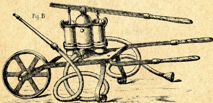
Pompe à deux corps aspirante & foulante
